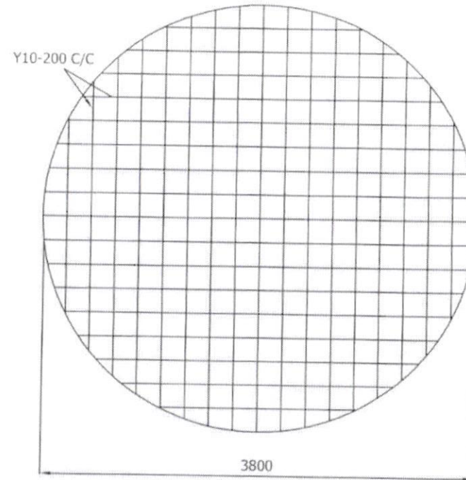
BOTTOM LAYER
