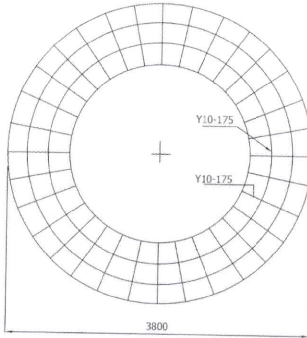
TOP LAYER
